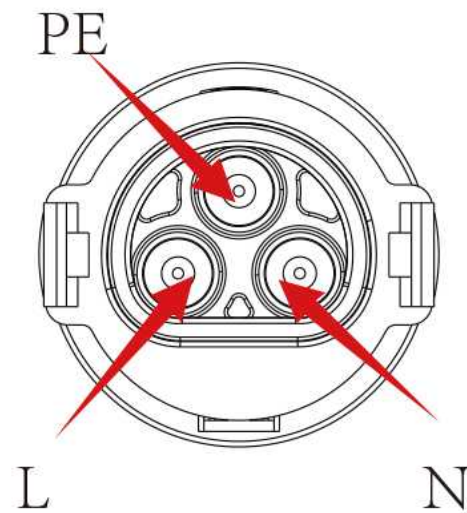
Steckverbinder
