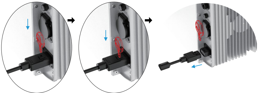
Zum Entriegeln des AC-Netzanschlusses.
